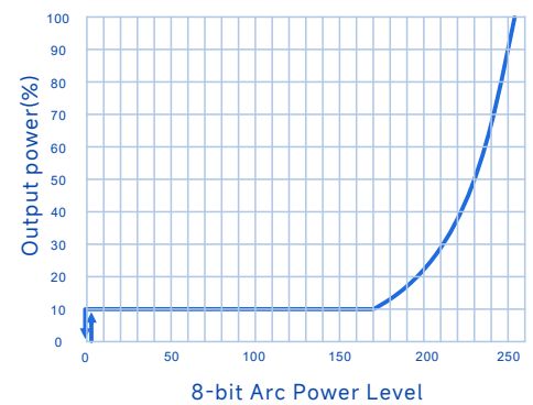
对数调光曲线
